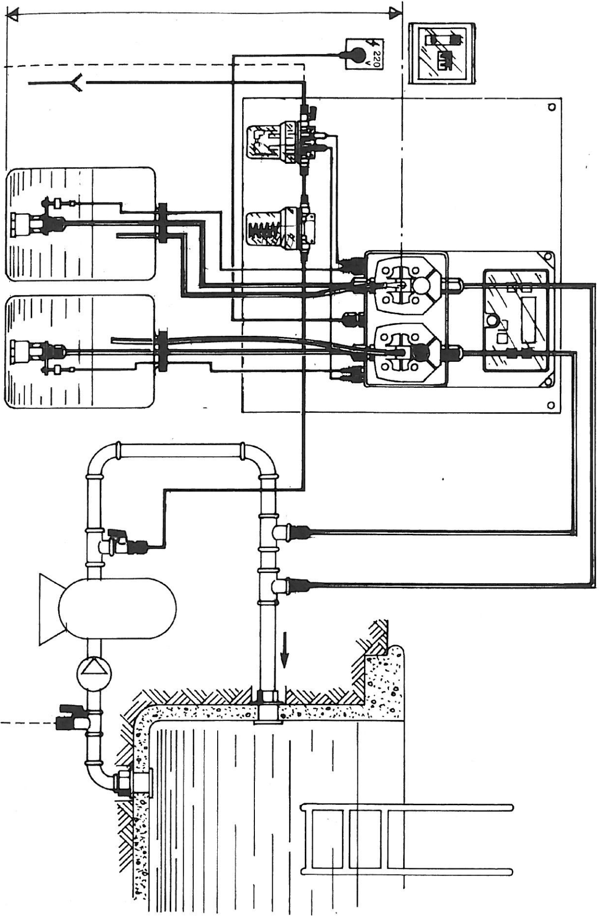
Anschlussbeispiel "DPHRHD"
