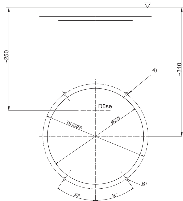
4) Befestigung an der Schalung (4x)
